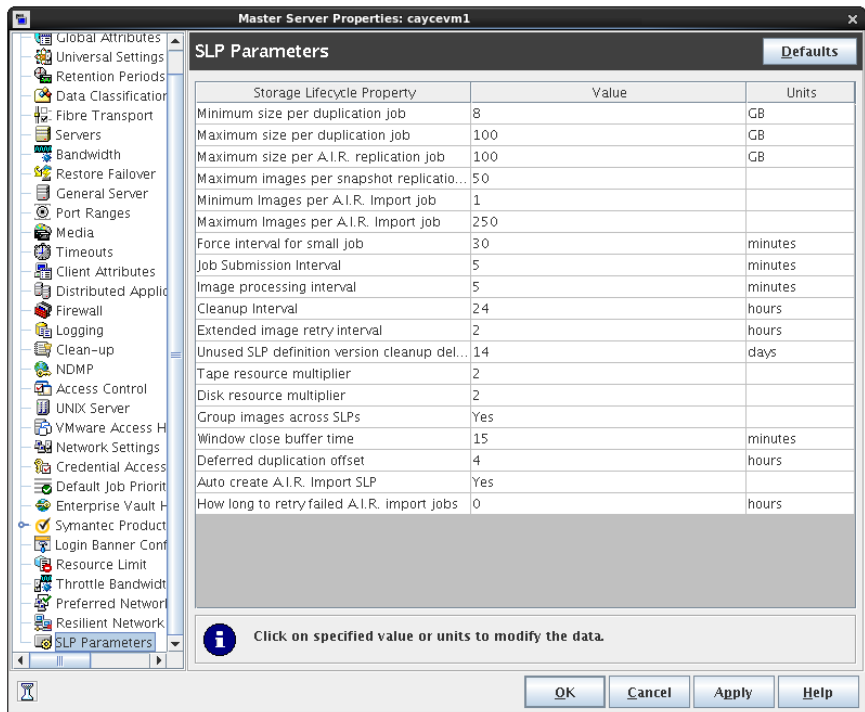
Figure 3-66 SLP Parameters dialog box
